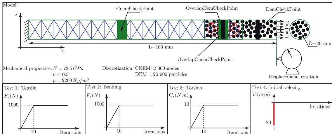
Fig. 18. Validation model.
