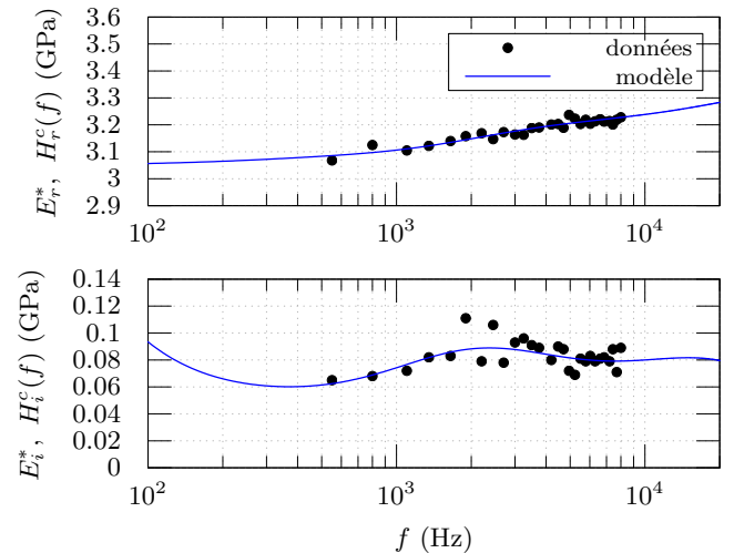
FIGURE 3 – Partie réelle (haut) et imaginaire (bas) des données expérimentales \{\omega_k, E_k^*\}_k [5] et de la réponse H^c(\omega) du filtre pour N_f = 4 .
