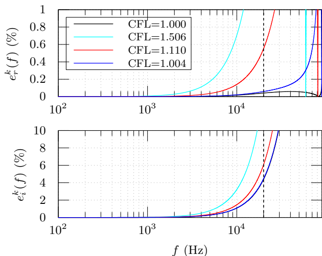
FIGURE 6 – Erreur sur la dispersion (haut) et la dissipation (bas) à CFL=1 (noir), CFL=1,004 (bleu), CFL=1,110 (rouge) et CFL=1,506 (cyan).
