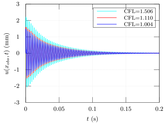
FIGURE 4 – Évolution temporelle u(x_{\text{obs}}, t) à CFL=1,004 (bleu), CFL=1,110 (rouge) et CFL=1,506 (cyan).
