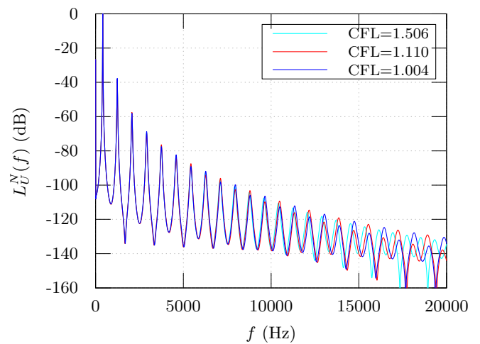
FIGURE 5 – Spectre du niveau de puissance L_U^N à CFL=1,004 (bleu), CFL=1,110 (rouge) et CFL=1,506 (cyan).
