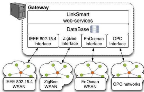
Fig. 2. Proxy scheme.
