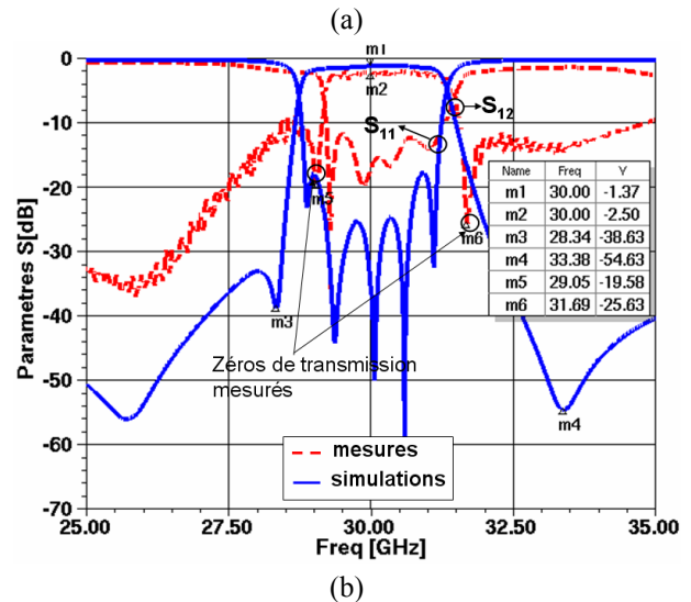
Figure 8. (a) Photo du filtre réalisé et (b) Performances électriques mesurées.
