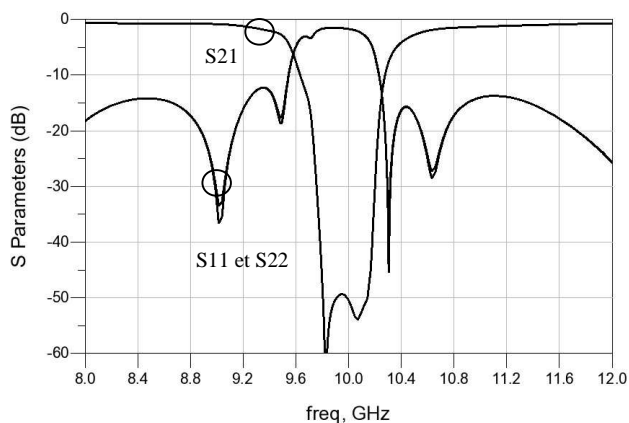
Figure 8. Simulation EM du filtre coupe-bande symétrique d'ordre 7
