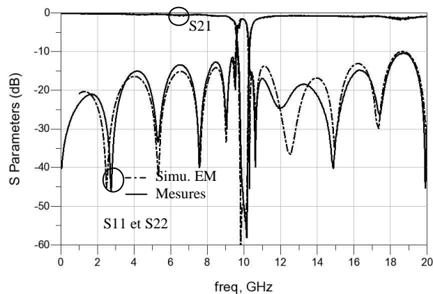
Figure 10. Simulation EM d'un filtre coupe-bande symétrique d'ordre 7
