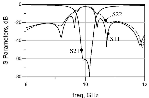
Figure 2. Simulation EM d'un filtre d'ordre 7 asymétrique
