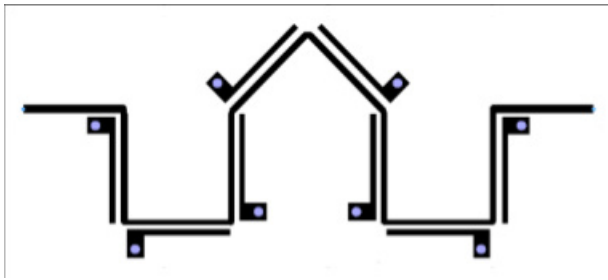
Figure 7. Masque du filtre coupe-bande symétrique d'ordre 7
