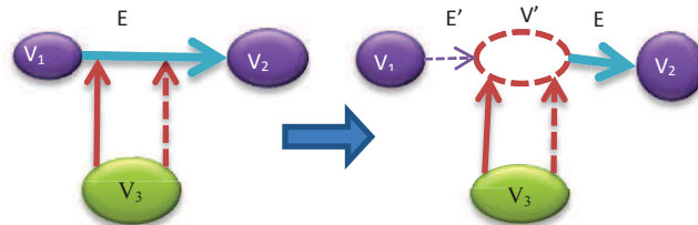
Figure 3. Lien sommet-Arête
