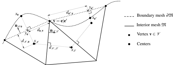
Fig. 1: Finite-volume meshes
