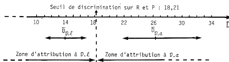
FIG. 11.— Discrimination quadratique de Diplectanum aequans ( D.a ) et Diplectanum laubieri ( D.l ). Les zones d'attribution à D.a et D.l (établies à partir des variables R et P considérées simultanément), les moyennes \bar{D} pour chacune des espèces (et les valeurs extrêmes observées de part et d'autre de ces moyennes) ont été représentées.
