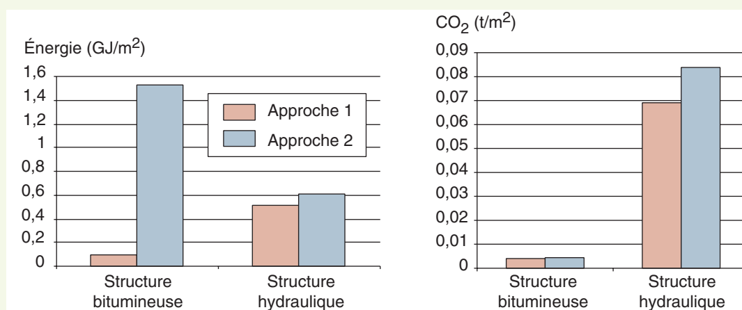
figure 2 Comparaison des indicateurs énergie et carbone pour les deux structures, selon les deux approches. Seules les contributions des constituants des mélanges de la chaussée sont prises en compte.
