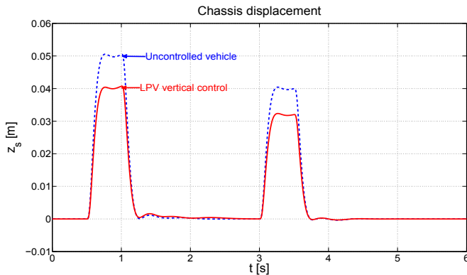
Fig. 9. Chassis displacement
