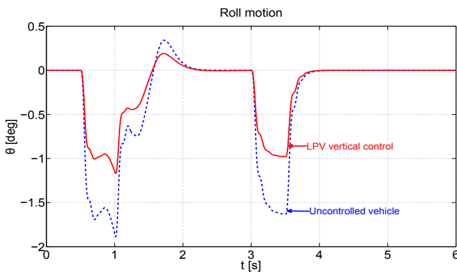
Fig. 10. Chassis displacement
