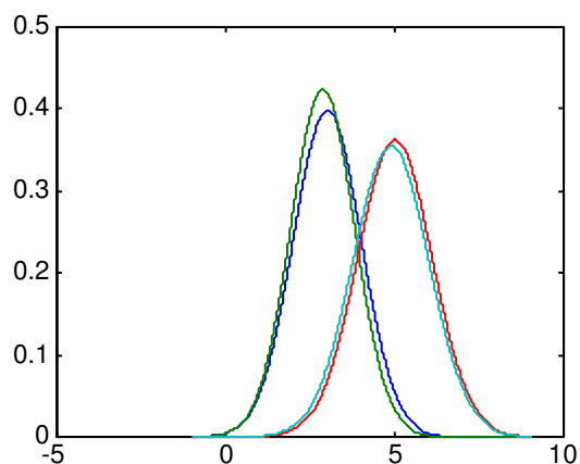
Figure 4 : Distributions théoriques et identifiées
