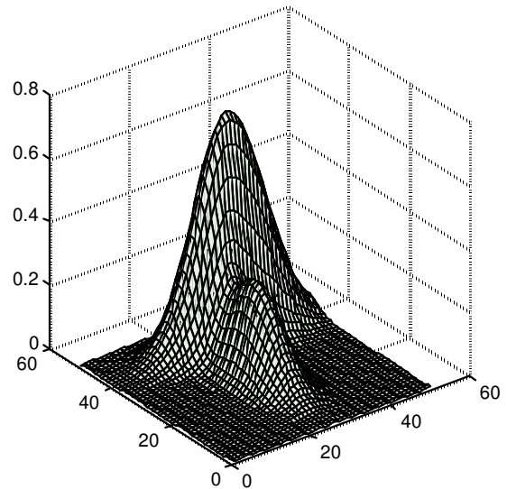
Figure 2 : Mélange de deux gaussiennes multi-variables
