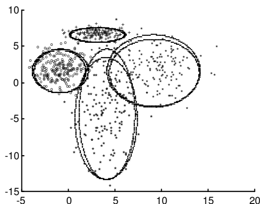
Figure 6 : Données et modèles identifiés
