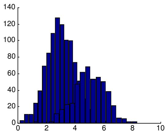
Figure 3 : Histogramme des deux distributions normales mono-variables
