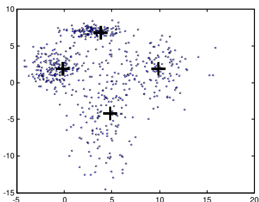
Figure 5 : Fonctions poids et allocation des données aux modèles locaux
