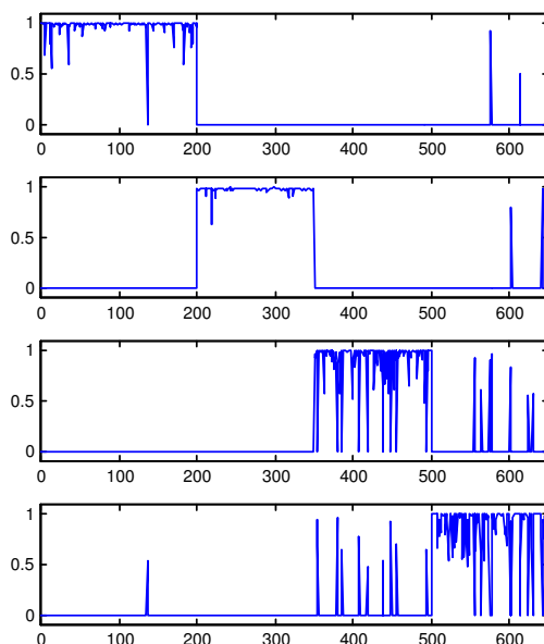
Figure 7 : Fonctions poids et allocation des données aux modèles locaux
