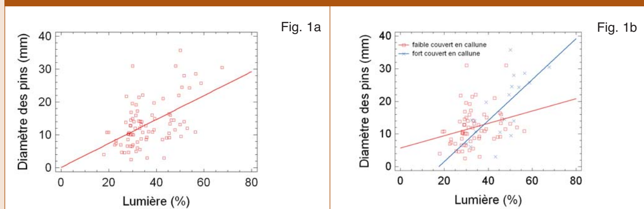
Figure 1 : Relation entre le diamètre des pins sylvestres et la disponibilité en lumière (éclairage direct + diffus) dans des trouées du massif de Lorris en forêt d'Orléans.
