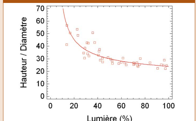
Figure 3 : Relation entre le coefficient d'élanement des semis de pin (rapport hauteur sur diamètre, H/D) mesuré en fin de première année et la lumière mesurée sous la callune, la molinie et la fougère (sans distinction d'espèces). Pépinière du Cemagref, Nogent/V
