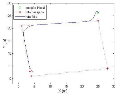
Figura 12. Respuesta del vehículo con relación al punto final.
