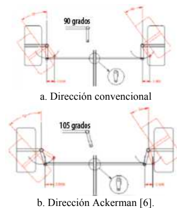
Figura 4. Configuración del sistema de dirección
