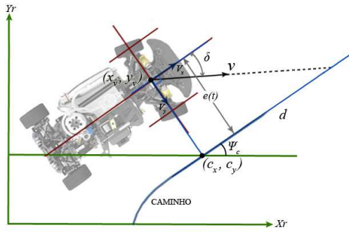
Figura 9. Análisis del error de orientación y localización.
