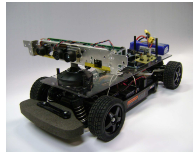
Figura 2. Vehículo Terrestre en escala Tamiya.
