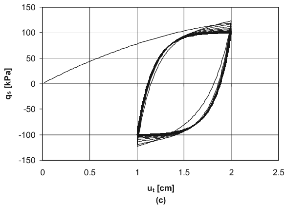
Figures 2. Modélisation d'essai de cisaillement suivant différentes conditions (a : déplacement symétrique, b : déplacement non symétrique – relaxation, c : déplacement non symétrique – relaxation nulle)
