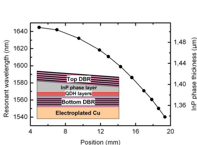
Fig.1- Variation de la longueur d'onde de résonance en fonction de la position sur l'échantillon (en insert le schéma de la cavité).
