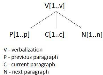
Fig. 1. Evaluation technique
