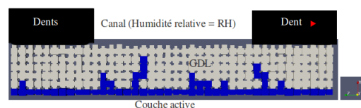
FIGURE 2 – Schéma du domaine de calcul
