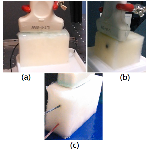
FIGURE 2 – Photographies des fantômes bi-modalités imagés. (a) Gaine en plastique noir moulée dans du cryogel, (b) inclusion sphérique de cryogel teinté à l'encre de Chine, le tout dans du cryogel, (c) tubes remplis d'encre noire ou vermillon, moulés dans du cryogel.
