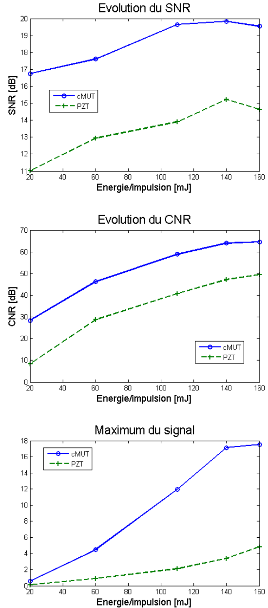
FIGURE 5 – Evolutions du SNR, du CNR et du maximum d'amplitude du signal en fonction des niveaux d'énergie pour les deux sondes.
