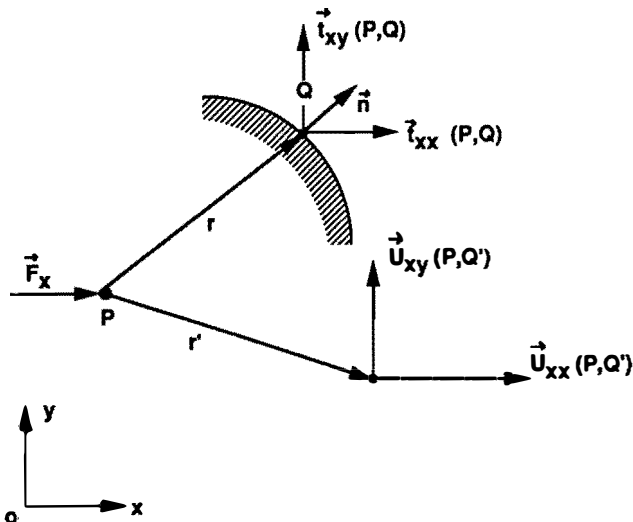
Fig. 2—Fundamental solution.
