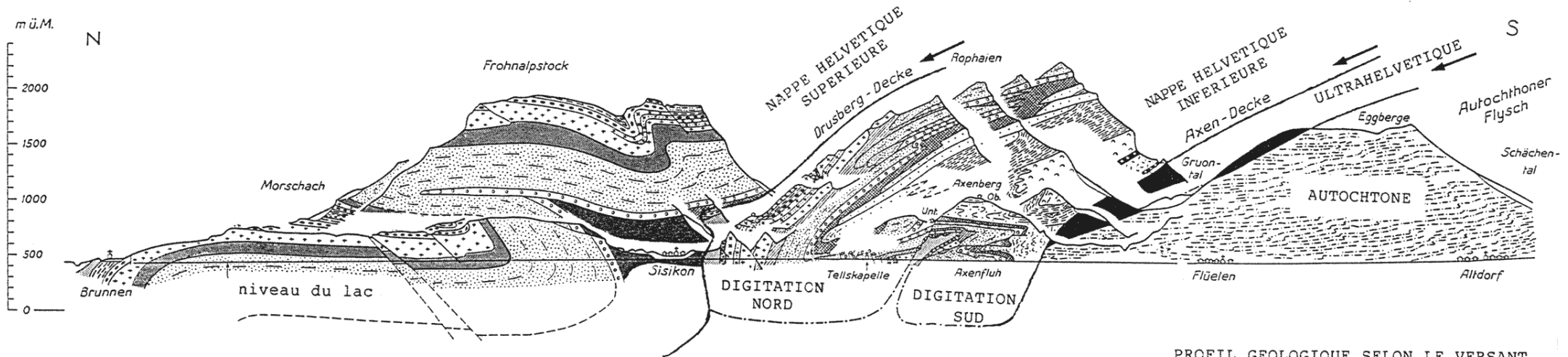
PROFIL GEOLOGIQUE SELON LE VERSANT EST DU LAC D'URI
