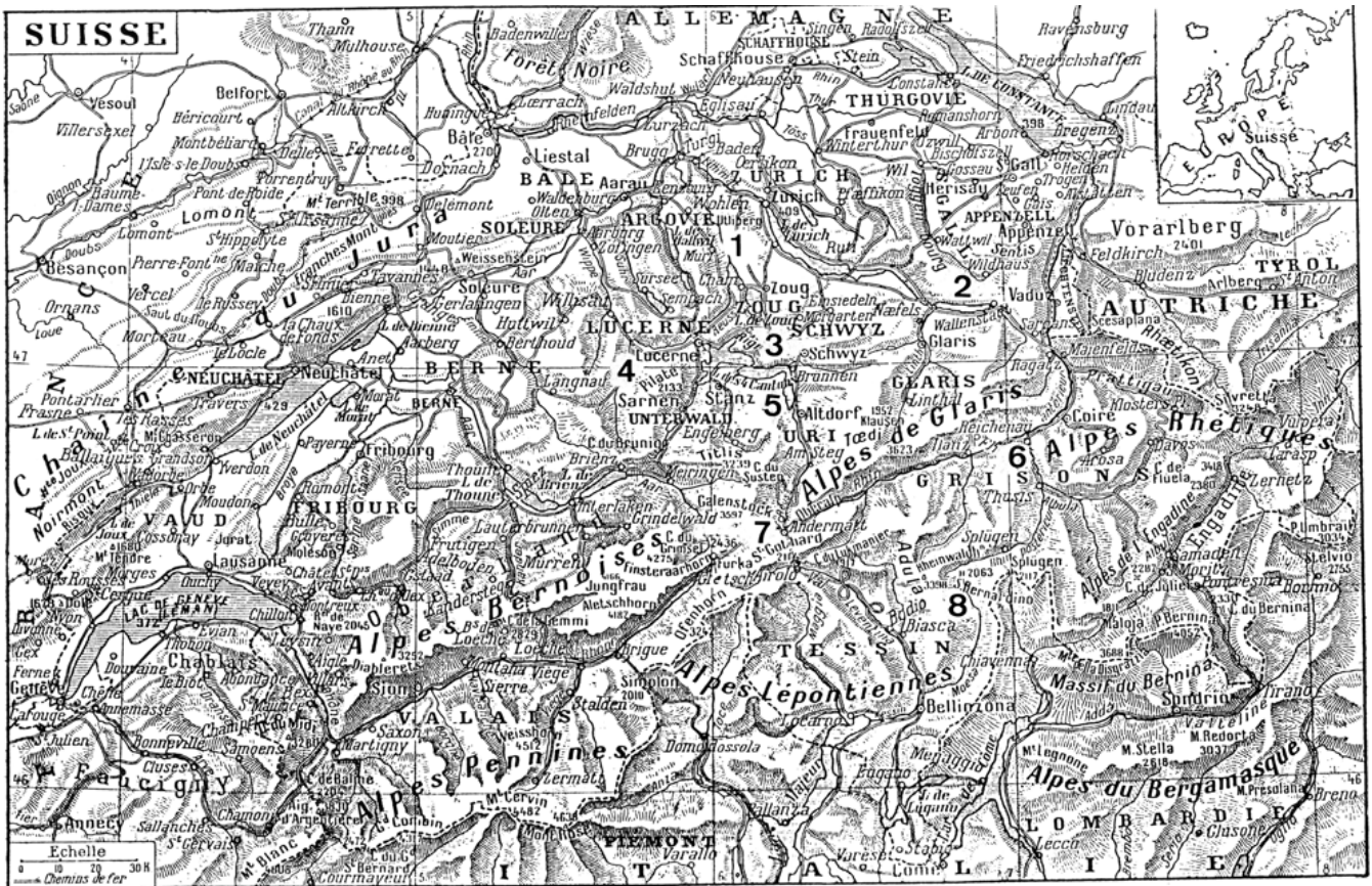
V - Carte sommaire de la Suisse, avec localisation des lieux mentionnés dans le texte de Johann Scheuchzer. - 1 Uttliberg; - 2 Wallensee ("lacus Rivarius"); - 3 Rigi; - 4 Pilatus; - 5 lac d'Uri; - 6 Via Mala; - 7 Saint-Gothard; - 8 Val Mesoccio.
