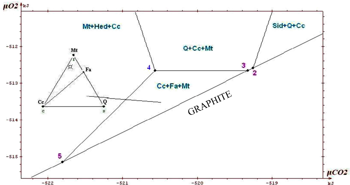
Figure 3a : Diagramme isotherme et isobare (600°C, 6Kb) \mu_{CO_2} - \mu_{O_2} des phases dans le système Ca-Fe-Si-C-O. Minerai Carbonaté 'Mc'.
