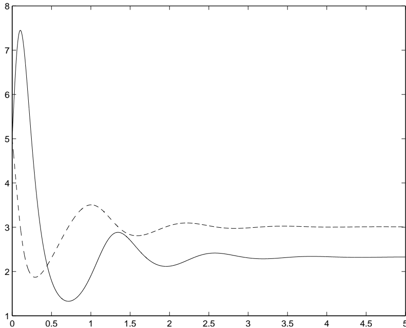
Figure 3.1: Dynamics of \rho (——) and I (---).
