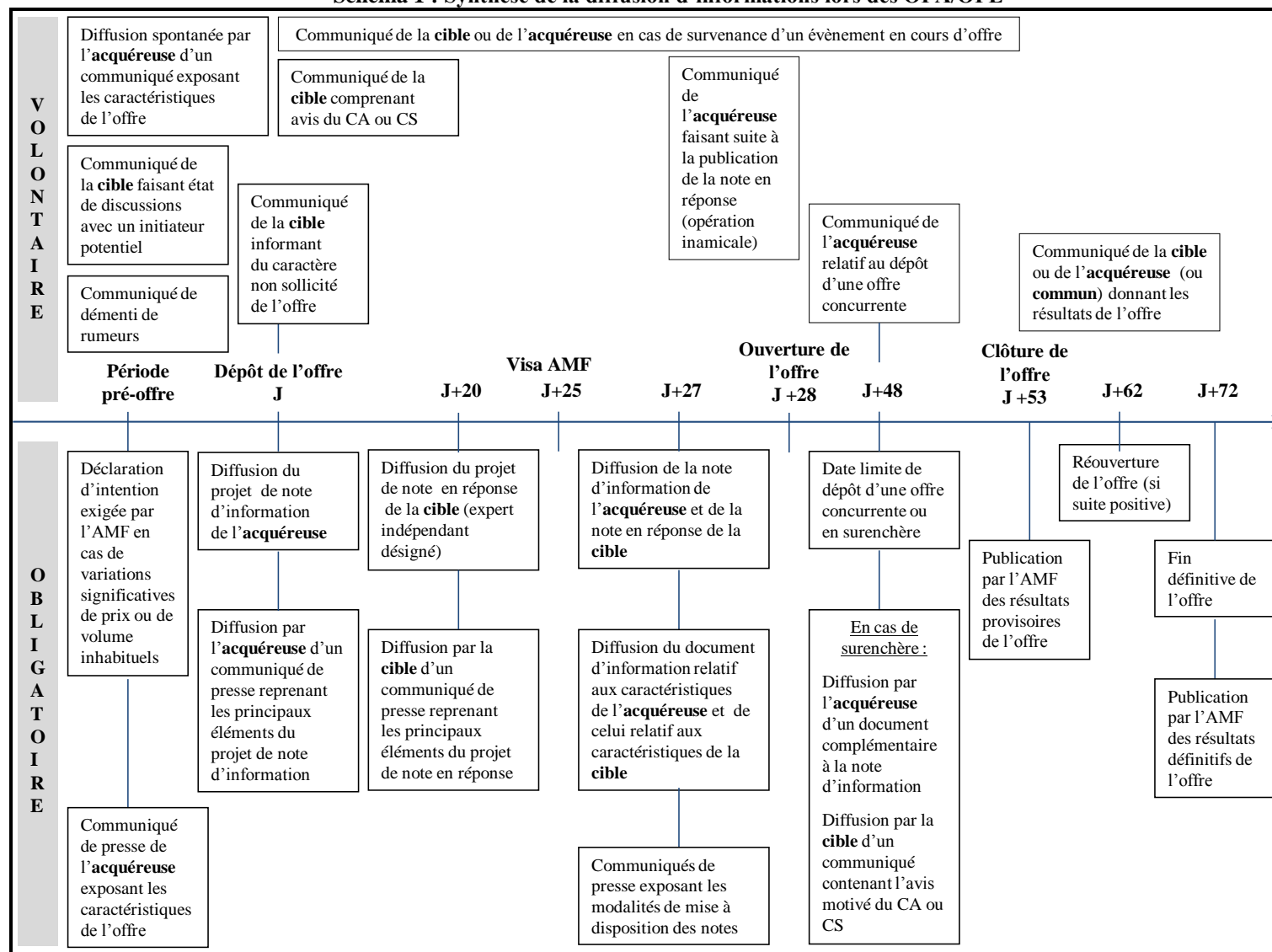
Schéma 1 : Synthèse de la diffusion d'informations lors des OPA/OPE
