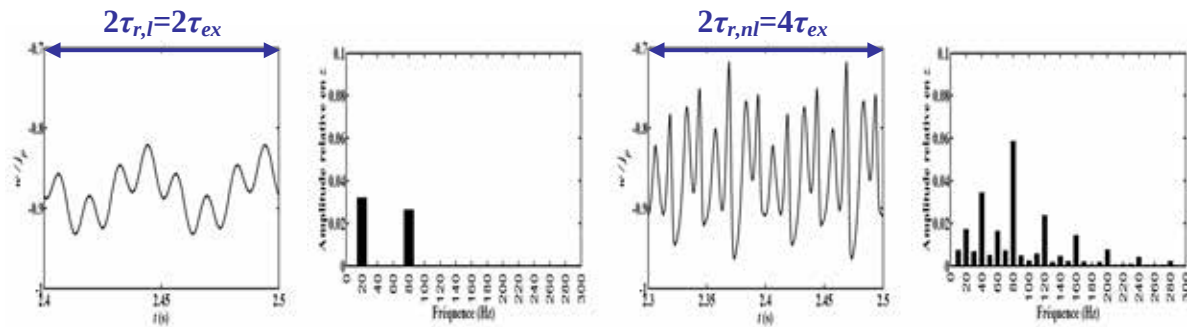
FIG. 5 – Réponses temporelles linéaire et non linéaire du rotor et leurs spectres au palier # 2 pour une rotation sinusoïdale du support d'amplitude \omega^{x,a} = 12 \times 10^{-2} rad/s et de fréquence \Omega^x = 80 Hz.
