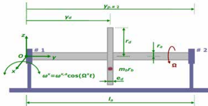
FIG. 2 – Diagramme schématique du rotor embarqué sur des paliers hydrodynamiques.
