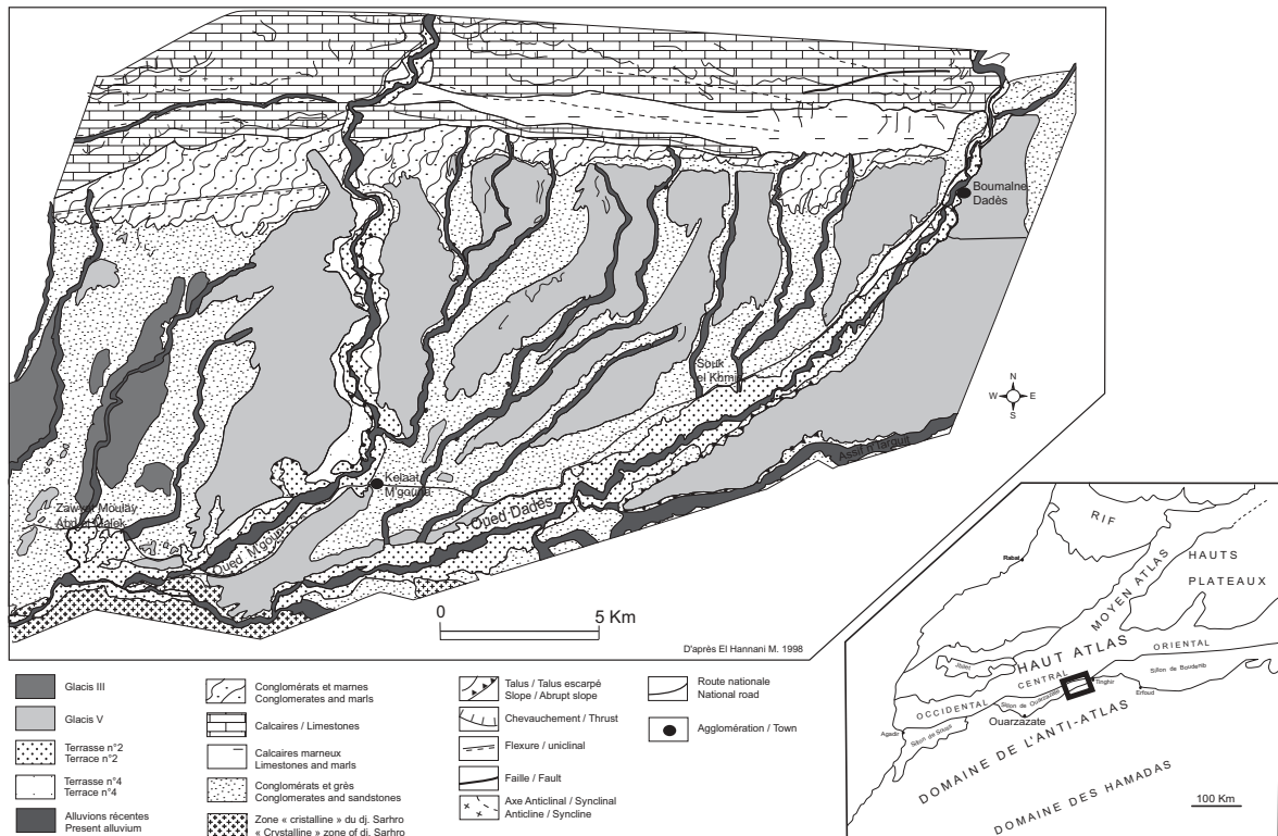
FIGURE 1 Cartes géomorphologique et de localisation de la zone est du bassin de l'oued Dadès. Geomorphological and location maps of the east part of wadi Dades basin.
