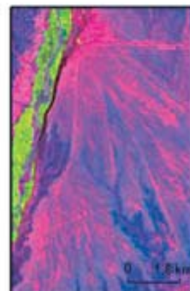
FIGURE 3 Composition colorée combinant trois axes d'une ACP sur les 6 canaux bruts TM de Landsat-5 du 27-08-1987. Axe 1 : bleu ; axe 3 : vert ; axe 2 : rouge. + 3 zooms. Color composite of three PCA axis using 6 TM Landsat-5 raw channels dated 27-08-1987. Axis 1 : blue; axis 3 : green; axis 2 : red. + 3 zooms.
