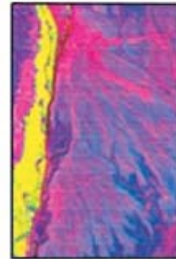
FIGURE 4 Composition colorée combinant trois axes d'une ACP sur les 6 canaux bruts TM de Landsat-5 du 05-03-1999. Axe 1 : bleu; axe 3 : vert; axe 2 : rouge + 3 zooms. Color composite of 3 PCA axis using 6 TM Landsat 5 raw channels dated 05-03-1999. Axis 1 : blue; axis 3 : green; axis 2 : red + 3 zooms.
