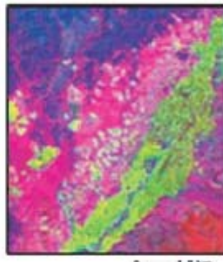
FIGURE 4 Composition colorée combinant trois axes d'une ACP sur les 6 canaux bruts TM de Landsat-5 du 05-03-1999. Axe 1 : bleu; axe 3 : vert; axe 2 : rouge + 3 zooms. Color composite of 3 PCA axis using 6 TM Landsat 5 raw channels dated 05-03-1999. Axis 1 : blue; axis 3 : green; axis 2 : red + 3 zooms.
