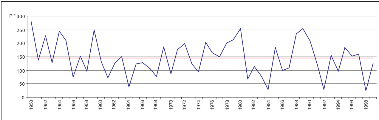
FIGURE 6 Variations inter-annuelles des précipitations par rapport à la moyenne (144,7 mm : 1950-1999). Inter-annual variations of rainfalls from the mean amount (144,7 mm : 1950-1999).
