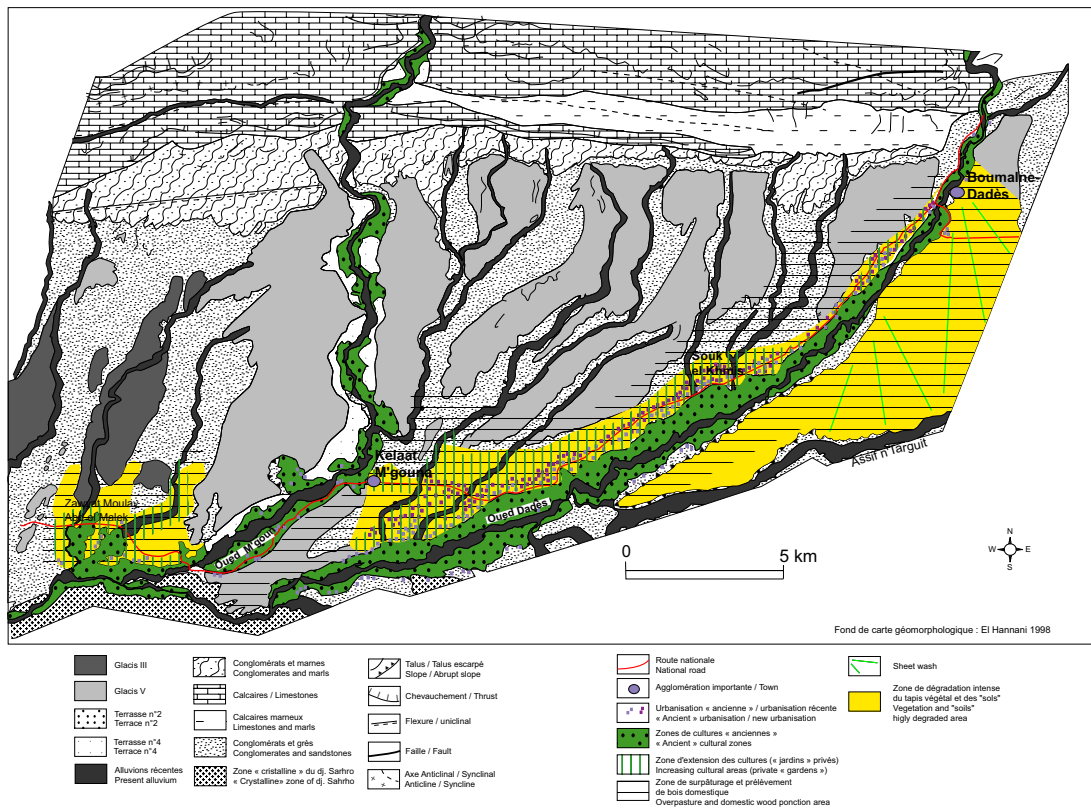
FIGURE 7 Croquis de synthèse des processus de dégradation et de leurs facteurs de la zone est du bassin de l'oued Dadès (Maroc). Degradation processes and factors synthetical sketchmap of the east part of wadi Dadès basin (Morocco).
