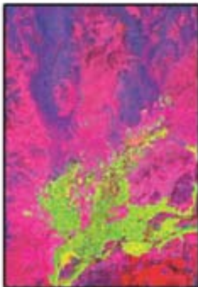
FIGURE 3 Composition colorée combinant trois axes d'une ACP sur les 6 canaux bruts TM de Landsat-5 du 27-08-1987. Axe 1 : bleu ; axe 3 : vert ; axe 2 : rouge. + 3 zooms. Color composite of three PCA axis using 6 TM Landsat-5 raw channels dated 27-08-1987. Axis 1 : blue; axis 3 : green; axis 2 : red. + 3 zooms.
