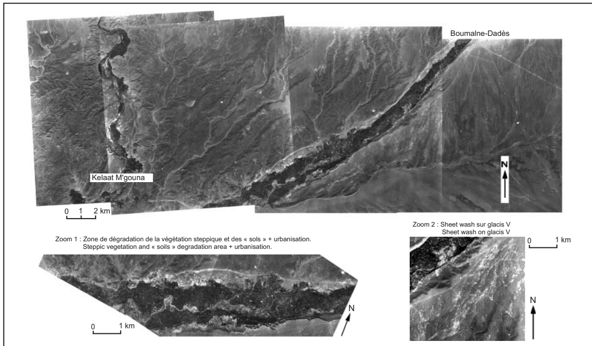
FIGURE 2 Mosaïque de photographies aériennes de 1964 : zone est du bassin de l'oued Dadès. Aerial photographs from 1964 : east part of wadi Dades.
