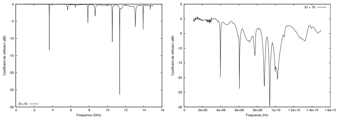
(a) Simulation : le premier mode de la structure s'établit à 3,665 GHz (b) Pratique : la première résonance se situe aux environs de 3,957 GHz
