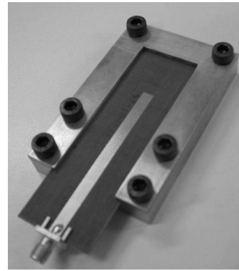
(a) Relevés de la fréquence de résonance. Les pertes du polymère élargissent le pic de résonance. (b) La structure de mesure montée. La carte de verre téflon avec la ligne microruban est insérée dans le support de laiton
