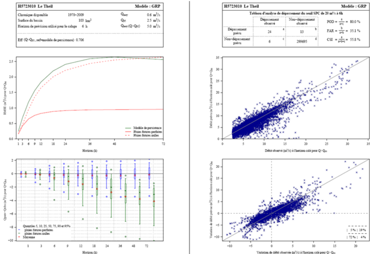
Figura 3: Exemplo da representação dos resultados do modelo GRP aplicado à bacia Theil (França). À esquerda um quadro com os detalhes da calibração realizada (nome e superfície da bacia, período da série de dados, horizonte de previsão e estatísticas dos dados de vazão observados). Os gráficos mostram a evolução do erro quadrático médio (RMSE) e a diferença entre os valores de vazão previstos e observados em função do horizonte de previsão, acima do limite de um nível de monitoramento Q_{vig} . À direita o quadro mostra os critérios relativos à ultrapassagem de níveis de alerta. Neste exemplo, o modelo prevê corretamente 80% dos eventos em que o nível excede o limite e a taxa de alertas falsos é de 35%. Os gráficos mostram os valores de vazão previstos em função dos valores observados (em cima) e as variações dos mesmos (em baixo), com as porcentagens correspondentes. Neste exemplo, 5% das previsões, representadas no quadrante esquerdo superior, correspondem aos equívocos em momentos de diminuição de vazão (previstas como aumento) e 4% aos equívocos inversos: previsões de aumento em instantes de diminuição da vazão.
