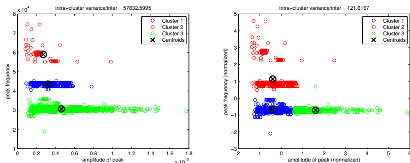
FIGURE 7 – Classification selon l’amplitude maximale et sa fréquence, avant et après normalisation
