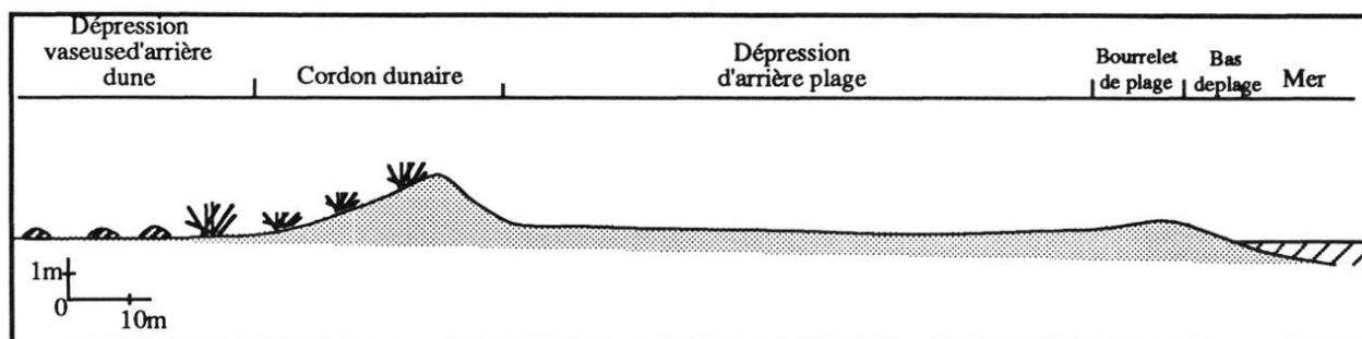
Fig. 1 - COUPE TRANSVERSALE DE LA PLAGE
