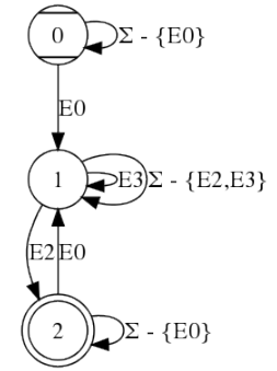
Fig. 5. Property 3 Automaton
