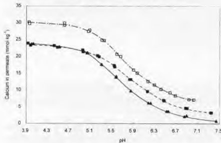
Fig 2. Solubilization with the pH at 20^\circ\text{C} of calcium from suspensions of native phosphocaseinate. Concentrations of calcium in permeates obtained by ultrafiltration on Centriflo CF25 are presented. The pH values were obtained after the addition of GDL during 15 h at 20^\circ\text{C} . Two replicates for each medium are presented. Same symbols as in the legend to figure 1. Solubilisation du calcium des suspensions de phosphocaseinate natif avec le pH à 20^\circ\text{C} . Les concentrations en calcium dans les perméats obtenus sur Centriflo CF25 sont présentées. Les différentes valeurs de pH étaient obtenues 15 heures après l'addition de la GDL à 20^\circ\text{C} . Deux répétitions de chaque suspension sont présentées. Mêmes symboles que pour la figure 1.
