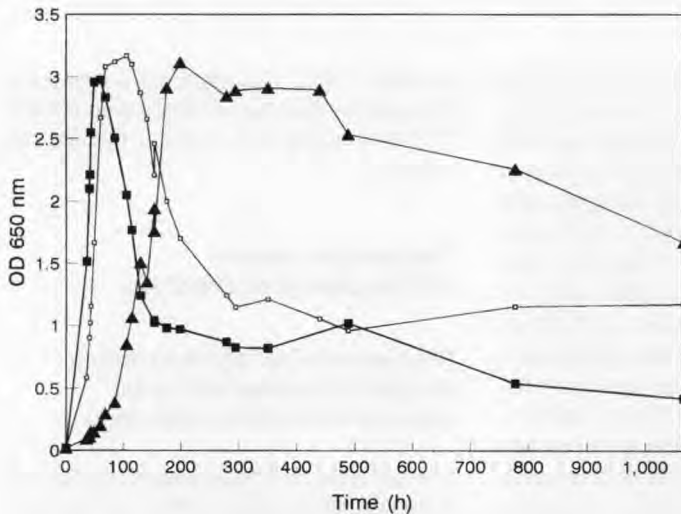
Fig 2. Growth of P. freudenreichii CNRZ 725 at different temperatures in YEL medium. Growth was followed by OD 650 for 1 100 h of incubation at 15°C (▲), 24°C (□) and 30°C (■). Croissance de P. freudenreichii CNRZ 725 en milieu YEL à différentes températures d'incubation. La croissance a été suivie par la mesure de la DO 650 sur une période de 1 100 h, pour 3 températures d'incubation : 15°C (▲), 24°C (□) et 30°C (■).
