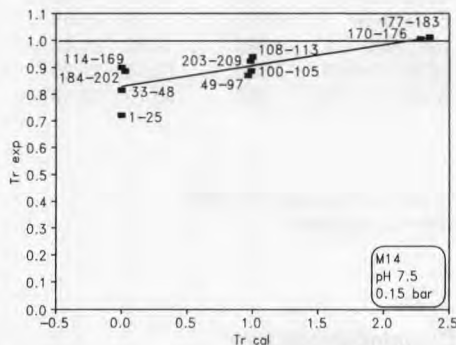
Fig 3. Experimental transmission, Tr_{exp} versus the predicted transmission calculated according to eq (7); Tr_{cal} ; peptides; M14 membrane. Transmission expérimentale, Tr_{exp} en fonction de la transmission calculée selon l'eq (7); Tr_{cal} : peptides, membrane M14.
