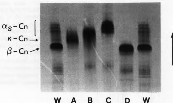
Fig 2. Alkaline PAGE (pH 8.9) in the presence of 4.5 mol/l-urea of whole caprine casein and fractions separated by RP-HPLC. W: whole casein; A: fraction A; B: fraction B; C: fraction C; D: fraction D. Électrophorèse en gel de polyacrylamide à pH alcalin en présence d'urée 4,5 mol/l de caséine entière caprine et des fractions séparées par HPLC. W: caséine entière; A : fraction A; B : fraction B; C : fraction C; D : fraction D.
