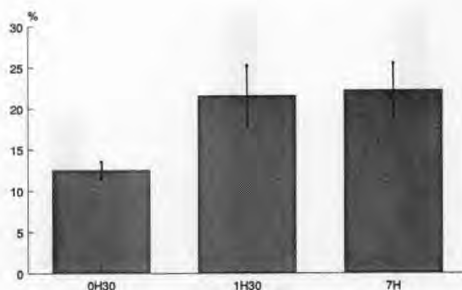
Fig 4. Emptied immunoreactive lactoferrin 30 min, 1.5 h and 7 h after the first meal in percentage of ingested lactoferrin with the first meal. Quantités de lactoferrine immunoréactive vidangées à 30 min, 1,5 h et 7 h de digestion, exprimée en % de la lactoferrine ingérée lors du premier repas.
