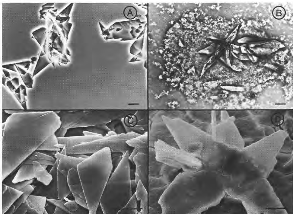
Fig 3. Morphologie des cristaux préparés en solution synthétique [A (40 x), C (8 000 x)] et du précipité obtenu après alcalination à pH 8,00, à 50 °C [B (40 x), D (8 000 x)]. Barre = 10 \mu m.
