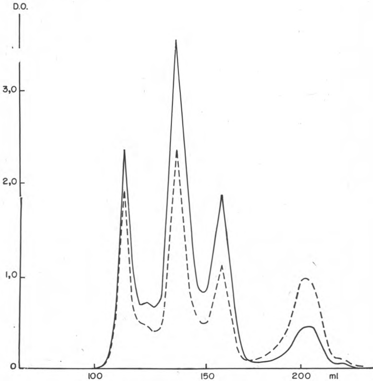
FIG. 4. — Filtration sur Séphadex G 100 de lactosérum de brebis (filtrat pH 4,5) Fractions de 10 ml — Vitesse de filtration 40 ml/heure. — Densité optique à 280 m \mu . ..... Densité optique à 260 m \mu .
