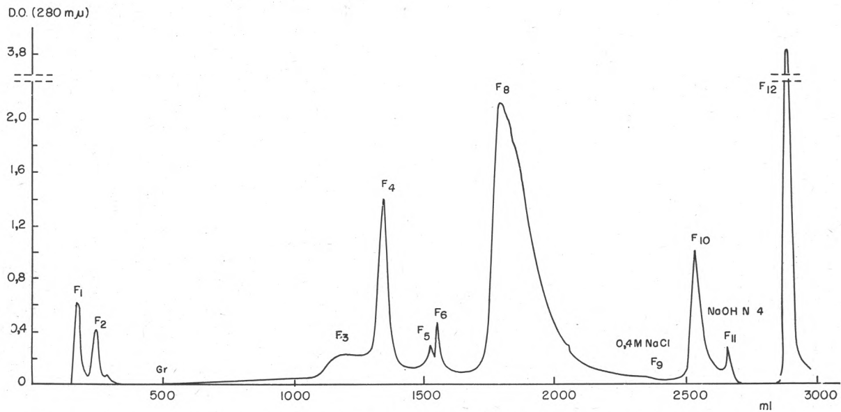
FIG. 1. — Chromatographie sur colonne de D.E.A.E.-cellulose de lactosérum individuel de brebis (filtrat pH 4,5)
