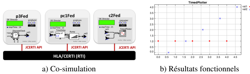
Figure 8. Fédération composée des 3 fédérés Ptolemy
