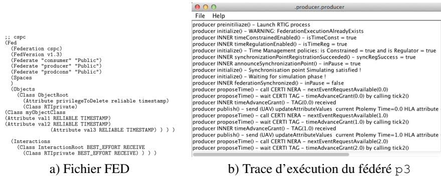
Figure 9. Observation des échanges entre Ptolemy et HLA/CERTI
