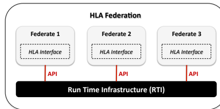
Figure 1. Architecture d'une fédération HLA
