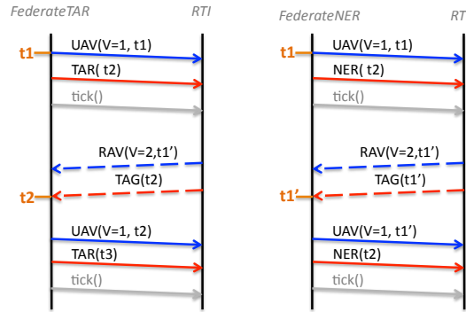
Figure 2. Services d'avancée temporelle : a. TAR b. NER
