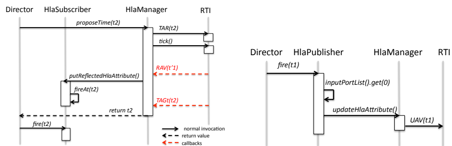
Figure 5. a. Avancement du temps
