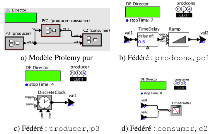
Figure 7. Eclatement d'un modèle Ptolemy centralisé en 3 fédérés
