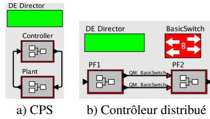
Figure 3. Modèles Ptolemy
