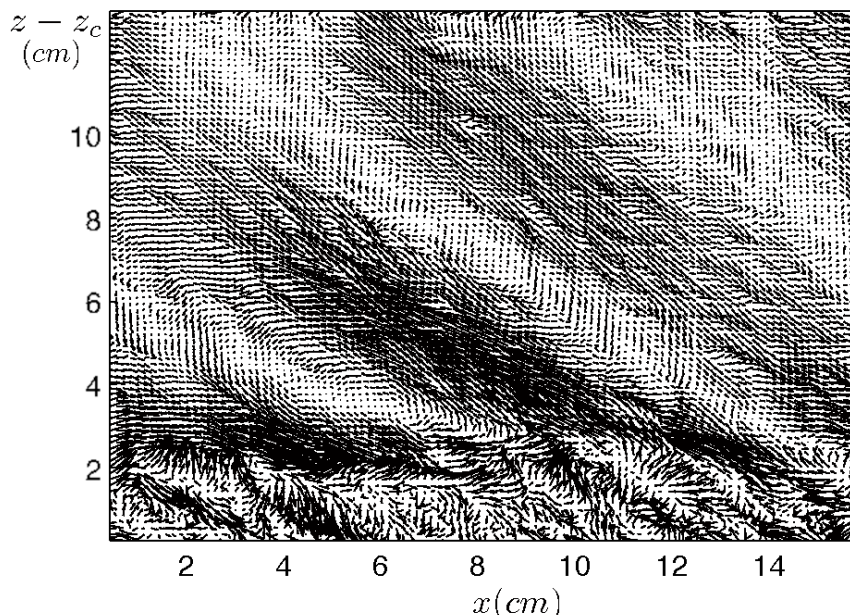
Figure 1: Champ de vitesse instantané mesuré par PIV dans la zone stratifiée. Seules les ondes se propageant vers la droite ont été gardées par notre processus de filtrage par Transformée de Hilbert.
