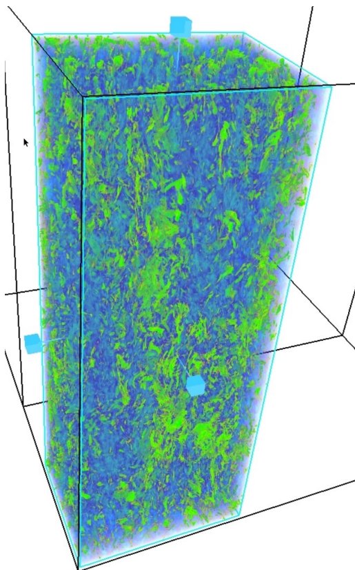
Figure 1: Simulation numérique directe ( 1024^3 point) d'une turbulence en rotation pour Ro=0.03 .
