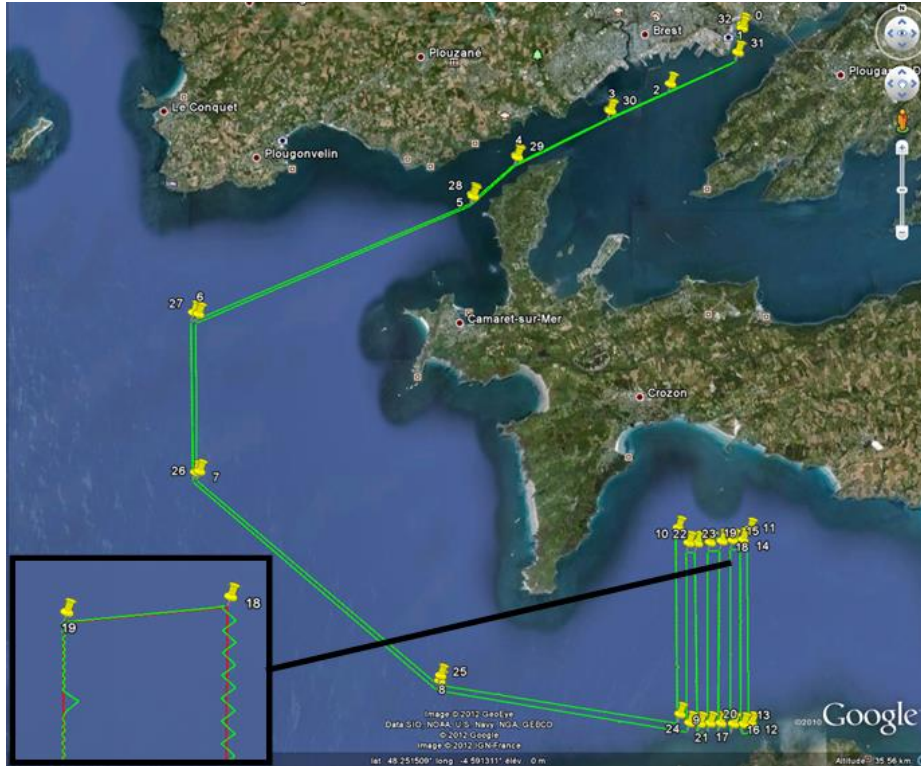
Figure 5 : Simulation de VAIMOS allant de Brest à Douarnenez. La trajectoire désirée (ligne rouge formée par les waypoints jaunes) et la trajectoire (simulée) effective (en vert) semblent superposées. Cependant, en zoomant, on s'aperçoit qu'il y a bien des phases de remontée au vent avec changements de bords. On peut aussi distinguer les étapes de recalibration du moteur de voile (toutes les 2 h), où le voilier dérive pendant une minute
