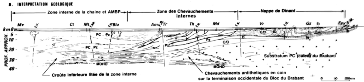
Fig. 4. Interprétation géologique du profil Nord de la France (ECORS Nord de la France, Ed. Technip 1988). Pour les abréviations forages et failles, voir les légendes des figures 2 et 3. AMBP = Anomalie magnétique du Bassin de Paris ; PC Précambrien ; Pz Paléozoïque ; C/O Cambro-Ordovicien ; D Dévonien ; H Houiller.
