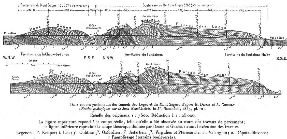
Fig. 1. Profils géologiques à travers le Jura neuchâtois (tunnels ferroviaires des Loges et du Mont-Sagne), établis par Amanz Gressly. La coupe théorique établie avant le percement (partie inférieure de la figure) a été confirmée lors des travaux (coupe réelle, partie supérieure de la figure) (Desor et Gressly, 1859). [La présente figure est reproduite d'après E. de Margerie (1922) : Le Jura , Fig. 70.]
