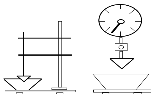
Figure 8 : Pénétromètres à chute libre : exemple d'un cône de Malher
