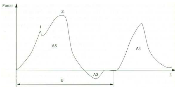
Figure 26 : Courbe type obtenue en profil de texture
