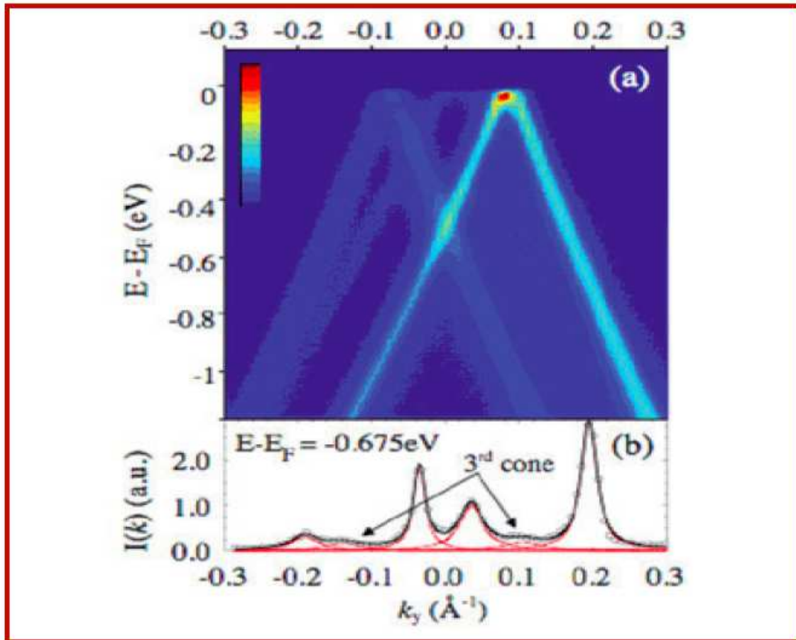
Figure 1 : (a) Structure de bande d'un film de graphène épitaxié d'une dizaine de couches sur 6H-SiC face carbone, mesurée par ARPES (intensité photoémise en fonction de l'énergie des électrons rapportée au niveau de Fermi E_F et de la direction d'émission ou vecteur d'onde). La température de l'échantillon est de 6 K, l'énergie des photons incidents est de 36 eV et la résolution en énergie est meilleure que 10 meV. Deux cônes linéaires sont bien visibles. (b) Coupe à E - E_F = -0,675 eV, montrant un troisième cône entre les deux premiers. Les trois cônes qui sont visibles proviennent des trois premières couches découplées de l'échantillon de graphène mesuré.
