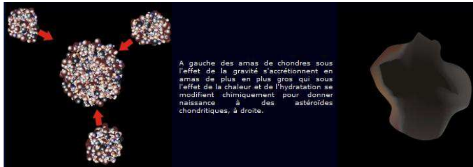
Figure 12 : Accrétion des astéroïdes chondritiques
