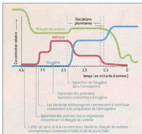
Figure 3 : Théorie récente d'évolution de l'atmosphère
