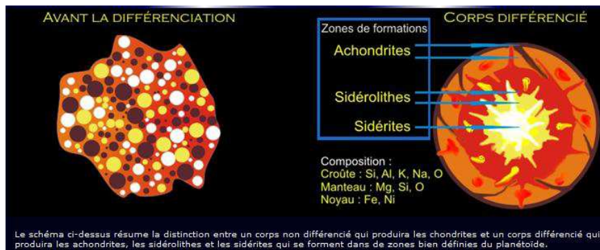
Figure 13 : Astéroïdes chondritiques et achondrites
