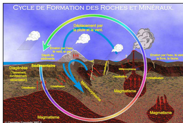
Figure 14 : Le cycle des roches
