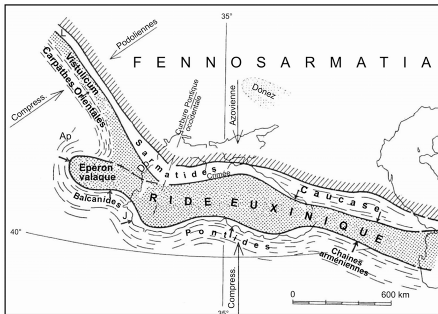
Fig. 7. L'éperon valaque et les Sarmatides dans l'avant-pays carpatique. Ap : Apusénides ; Dd : Dobroudja ; J :Mons d'Istrandja (Strandja) ; L : Lysagora. Les petites flèches marquent les vergences principales (d'après Hans Stille, 1953, fig. 26).
