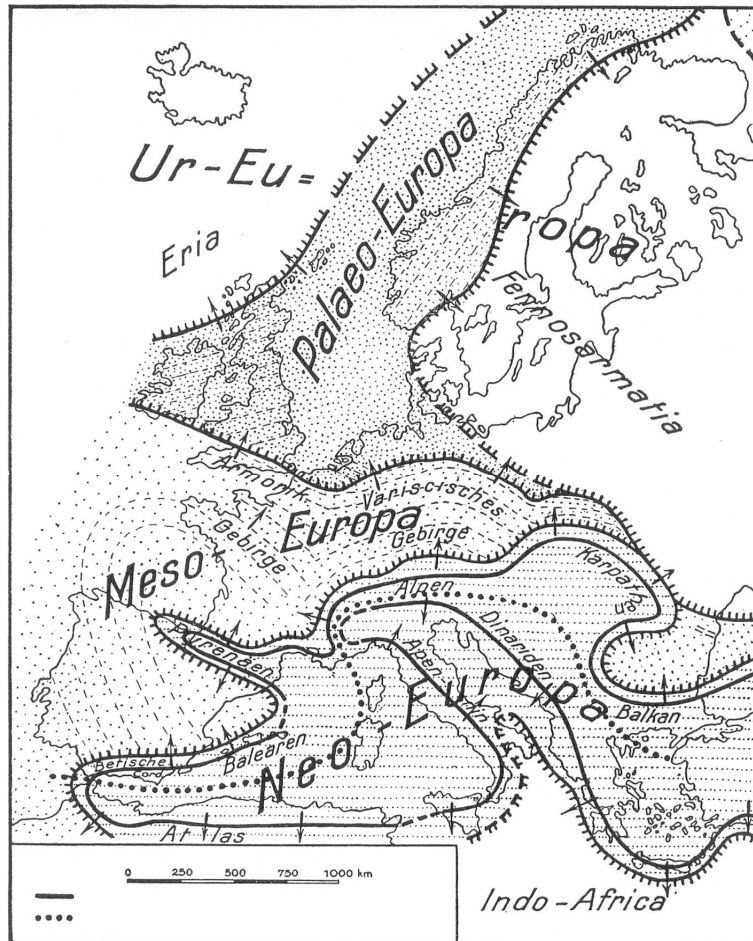
Fig. 3. Divisions géotectoniques de l'Europe et de l'océan Atlantique (d'après Hans Stille, 1924).
