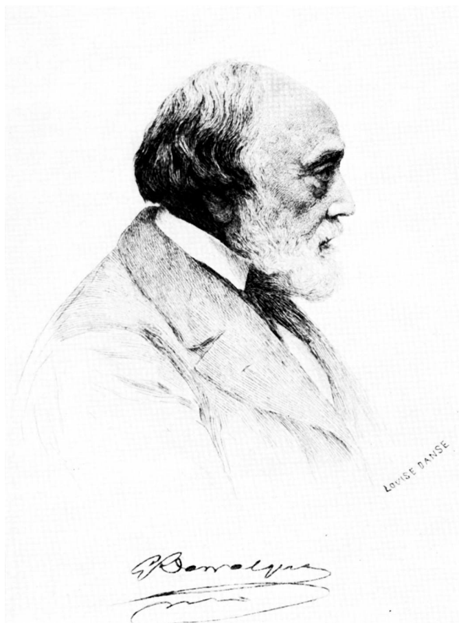
Fig. 4. Gustave Dewalque (1828-1905). Successeur d'André-Hubert Dumont à la chaire de géologie de l'université de Liège, il publie une longue liste de travaux dans les différents domaines des sciences minérales et fonde en 1873 la Société géologique de Belgique.
