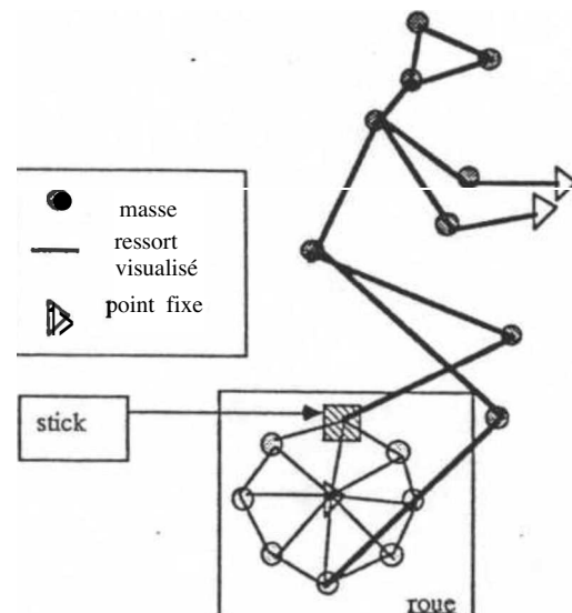
figure 5 - Modèle d'une structure de contrôle
