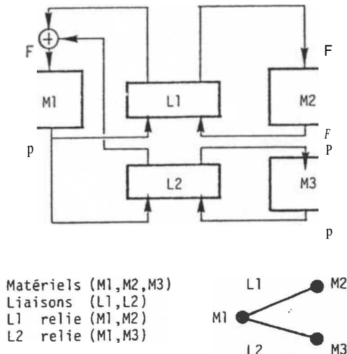
Figure 6 - Combinaison d'éléments mécaniques
