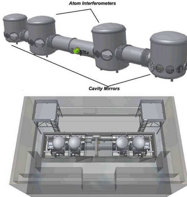
Fig. 30. – Design of the 10 m baseline MIGA-prototype at LP2N (Laboratoire Photonique Numerique et Nanosciences) in Bordeaux.
